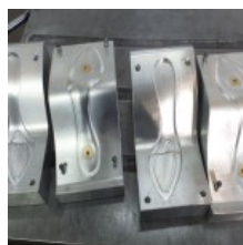
Stampo per fondi in polistirolo
